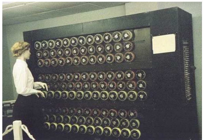
Bombe électromécanique
